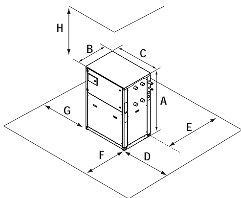
Unità interna
