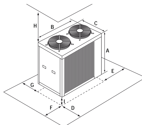
Außengerät
